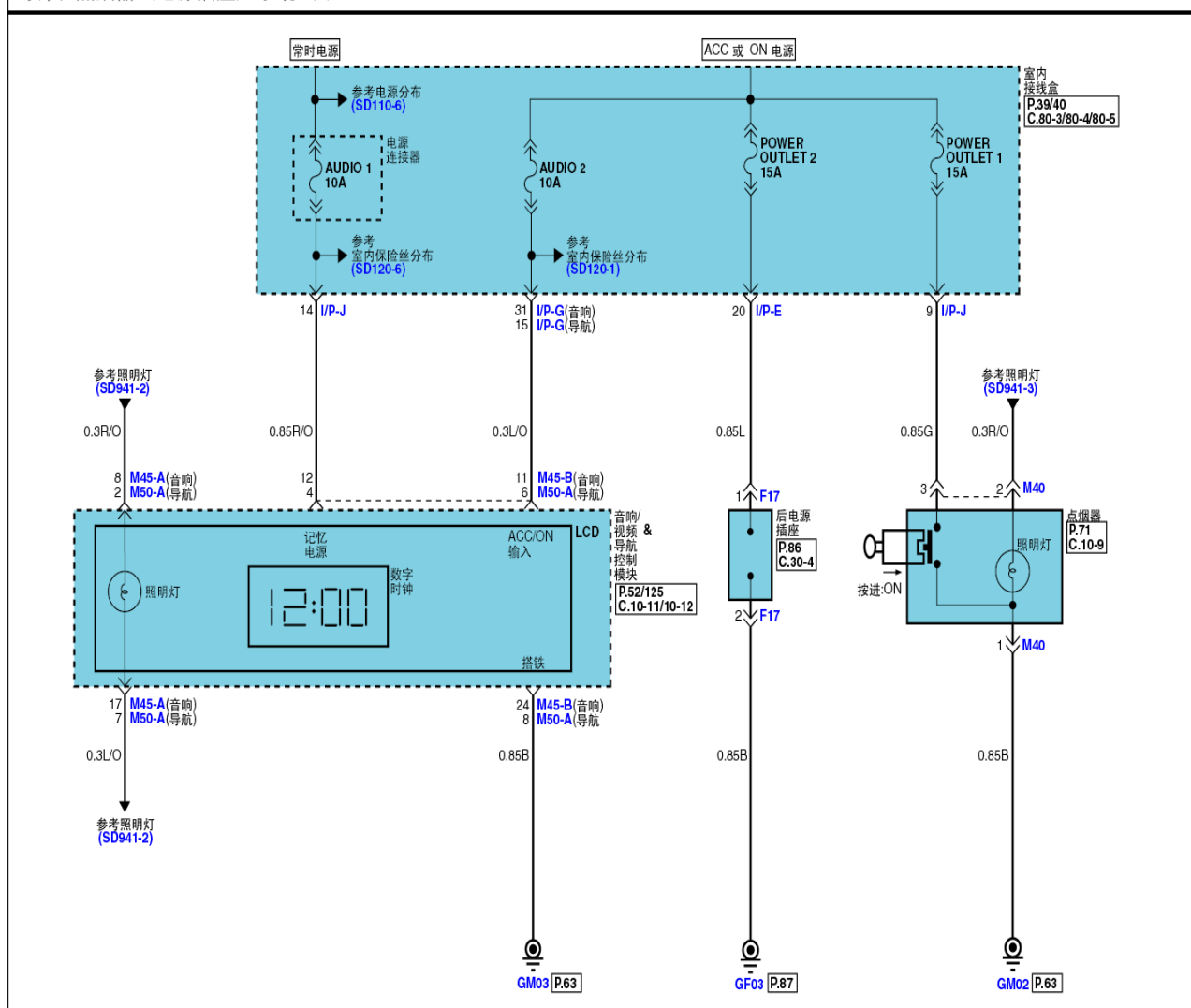
时钟和点烟器（电源插座）系统 (1)
